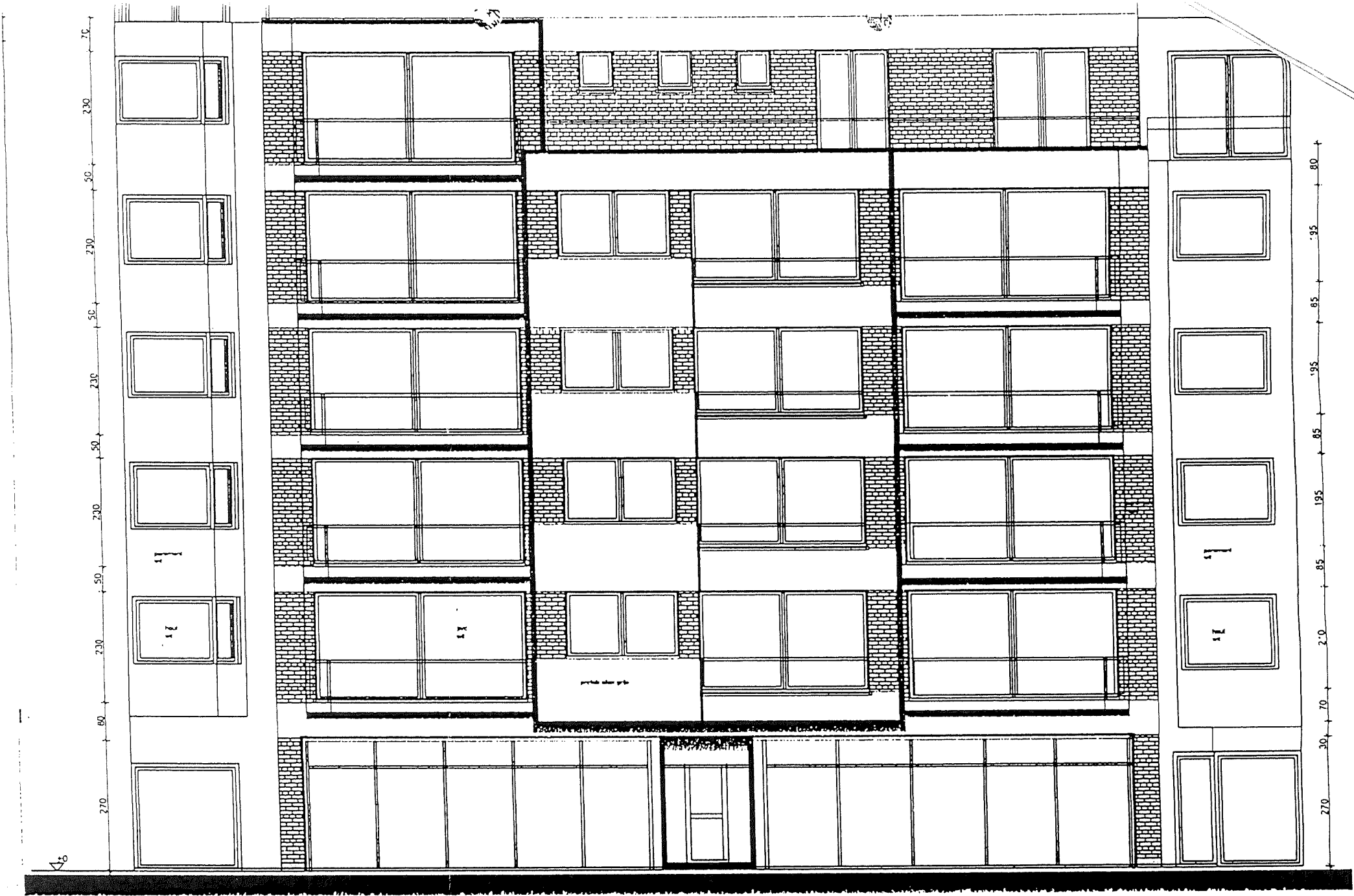
voorgevel
